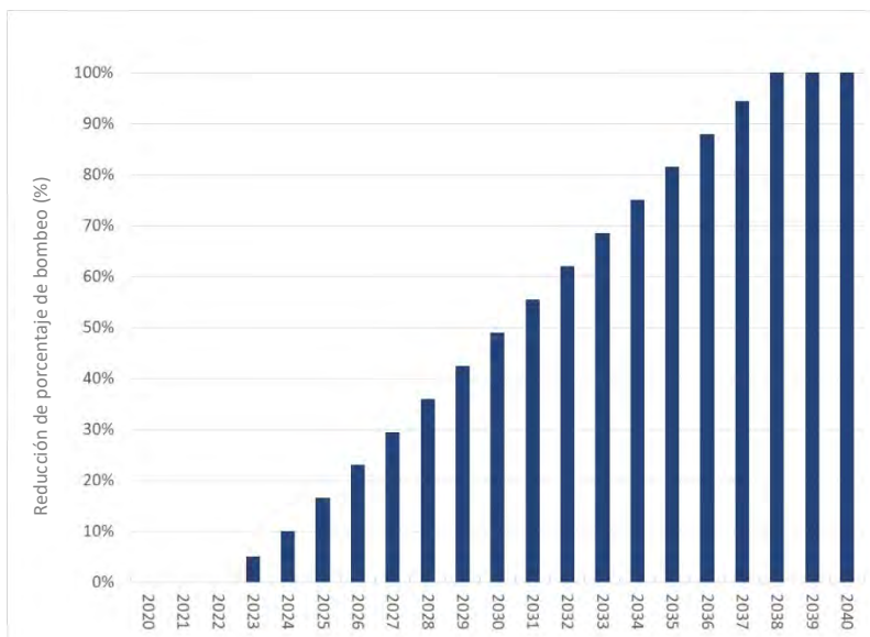
Figura ES-15: Programa de reducciones de bombeo de aguas subterráneas propuestas
